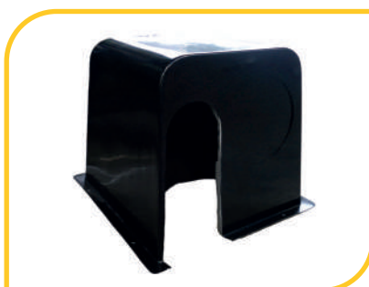
Coffrage insonorisation Dim. : 0,75 x 0,75 x h 0,62 m Prix : 255 €
